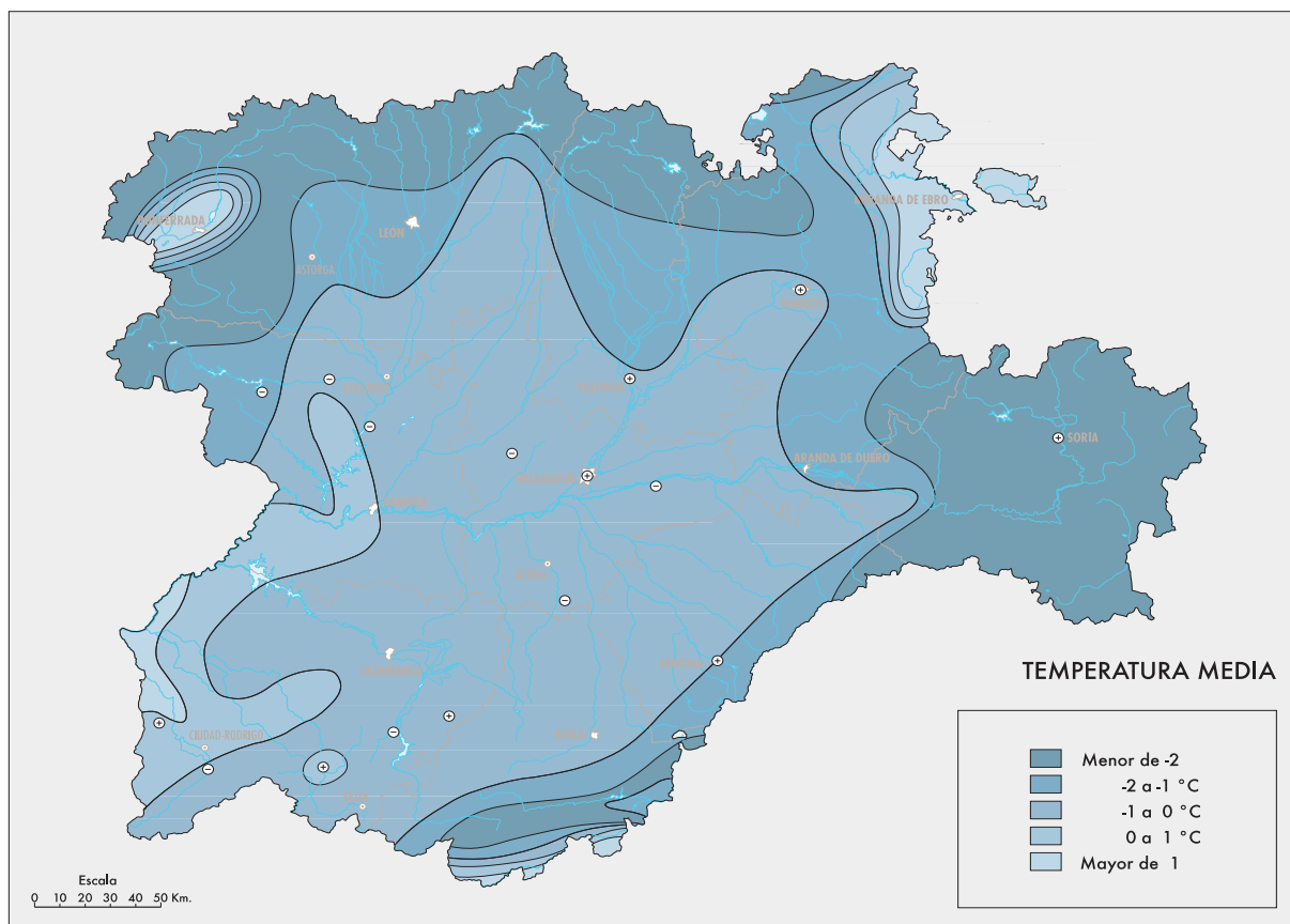
FIGURA 3.4 Mapa temperatura media mínimas de enero
